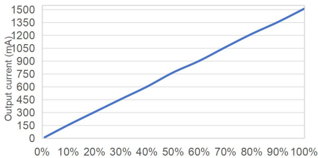
Linear dimming
