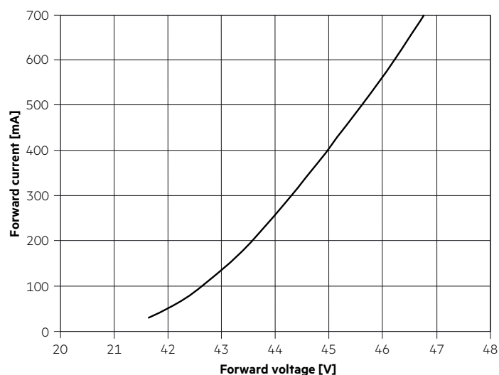
LLE 24x560mm 2400lm 8xx HV ADV6
